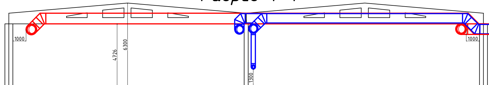
Разрез 4-4
